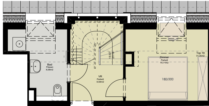
2. Dachgeschoss
