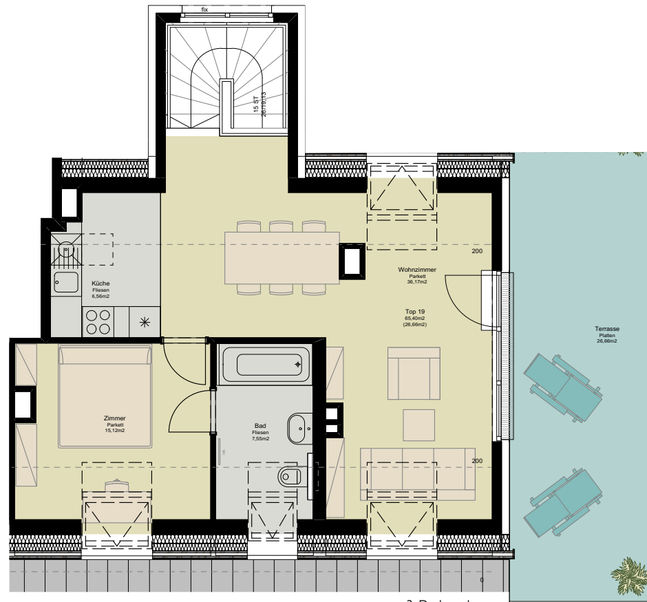
3. Dachgeschoss
